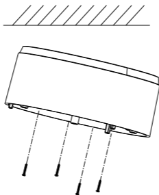
Figura 2-9 Instalați baza de montare
