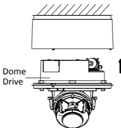
Figura 2-3 Instalați mecanismul de acționare al cupolei
