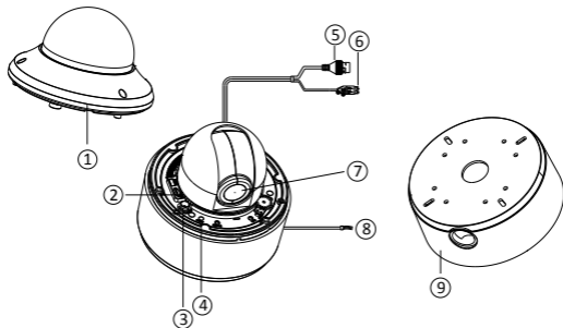
Figura 1-3 Prezentarea camerei de tip II dome
