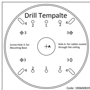
Figura 2-8 Șablonul de găurire
