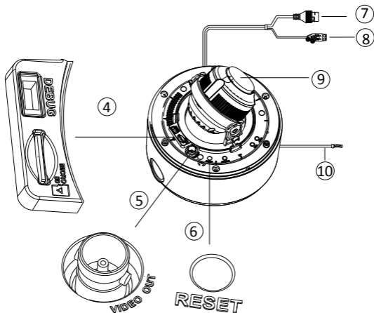
Figura 1-2 Prezentarea (2) camerei de tip II dome
