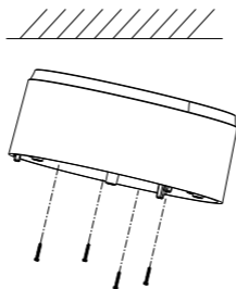
Figura 2-2 Instalați baza de montare
