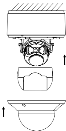
Figura 2-6 Instalați căptușeala neagră și bula
