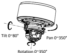
Figura 2-4 Reglare pe 3 axe
