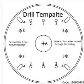
Figura 2-1 Șablonul de găurire
