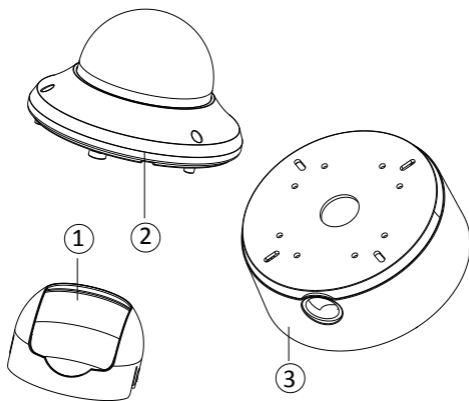
Figura 1-1 Prezentarea (1) camerei de tip I dome
