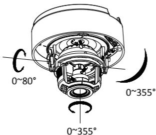
Figura 2-5 Reglare pe 3 axe
