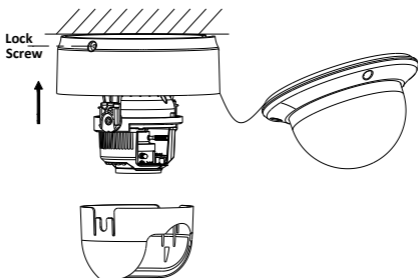
Figura 2-4 Instalați baza de montare
