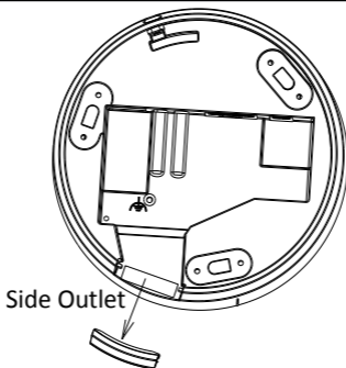
Figura 2-2 Orificiu de ieșire lateral
