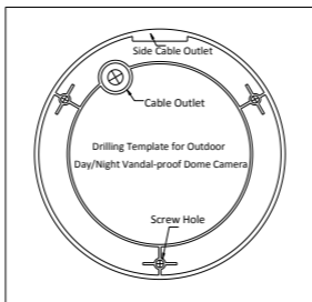
Figura 2-2 Șablonul de găurire
