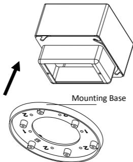
Figura 2-8 Montarea încastrată în tavan
