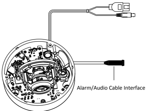
Figura 1-2 Interfață audio și de alarmă
