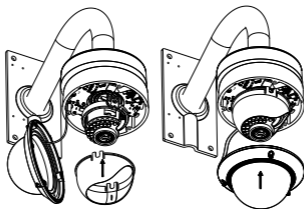
Figura 2-13 Fixați căptușeala neagră și bula
