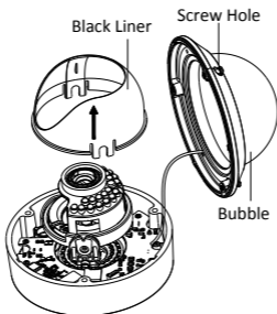
Figura 2-1 Scoateți bula și căptușeala neagră
