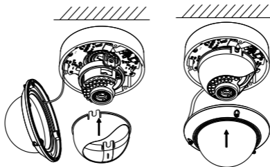
Figura 2-4 Fixați căptușeala neagră și bula
