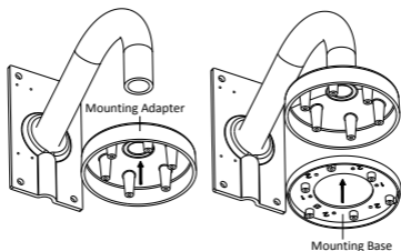
Figura 2-11 Instalați baza de montare
