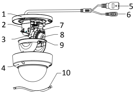
Figura 1-1 Prezentarea camerei tip I
