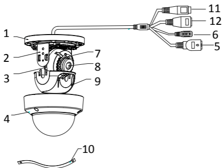
Figura 1-2 Prezentarea camerei tip II
