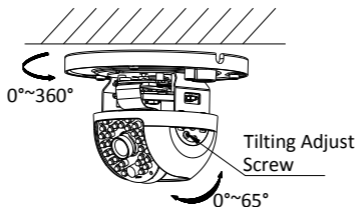
Figura 2-5 Reglarea unghiului la camera tip I
