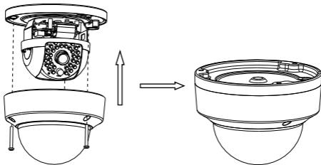
Figura 2-7 Reinstalarea bulei
