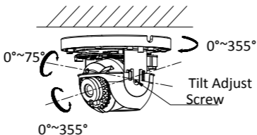
Figura 2-6 Reglarea pe 3 axe a camerei tip II.
