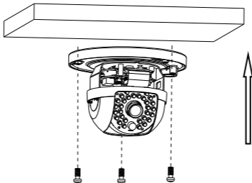
Figura 2-3 Fixați baza de montare
