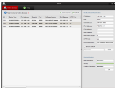
Figura 3-4 Interfața SADP
