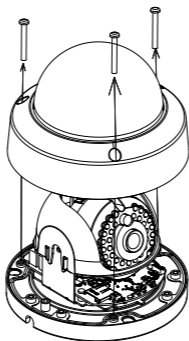
Figura 2-8 Demontați camera
