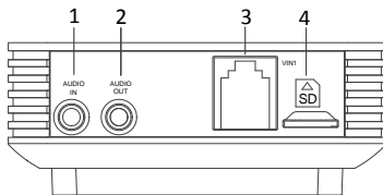
Figura 1-2 Panoul frontal de tip I
