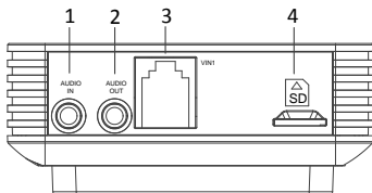
Figura 1-3 Panoul frontal de tip II
