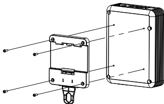
Figura 2-2 Fixați consola pe unitatea principală
