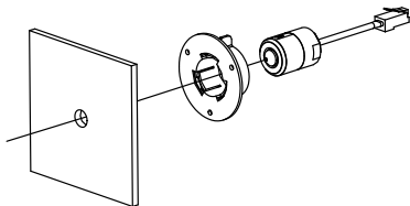
Figura 2-11 Instalați senzorul cilindric
