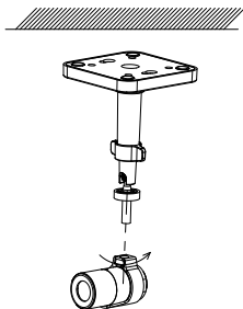
Figura 2-16 Instalați unitatea focală fixă pe consolă
