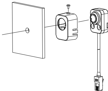
Figura 2-6 Introduceți unitatea de senzor în formă de bloc
