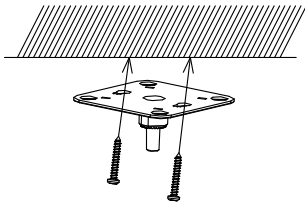
Figura 2-12 Fixați consola de montare pe tavan
