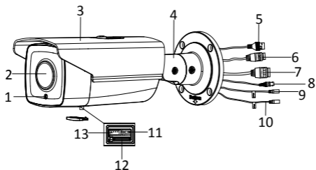
Figura 1-1 Prezentare
