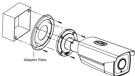
Figura 2-7 Montarea cu o doză de perete
