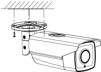
Figura 2-2 Instalați camera
