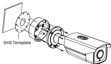
Figura 2-6 Instalarea cu o cutie de racord
