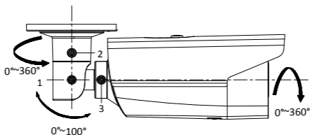
Figura 2-3 Reglați unghiul de supraveghere
