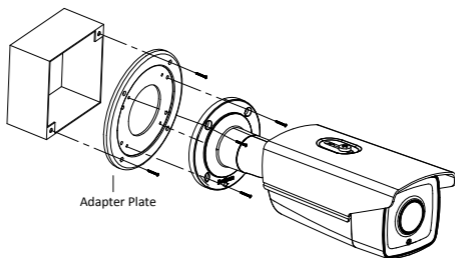
Figura 2-7 Montarea cu o doză de perete
