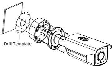
Figura 2-6 Instalarea cu o cutie de racord
