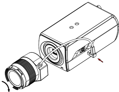
Figura 2-2 Instalați obiectivul
