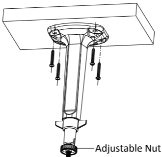
Figura 2-1 Instalați suportul
