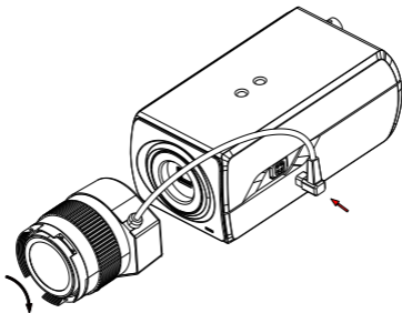
Figura 2-4 Instalați obiectivul
