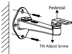
Figura 2-5 Instalați consola pentru perete
