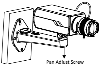
Figura 2-6 Instalați camera pe consolă
