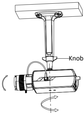
Figura 2-3 Instalați camera pe suport și reglați unghiul
