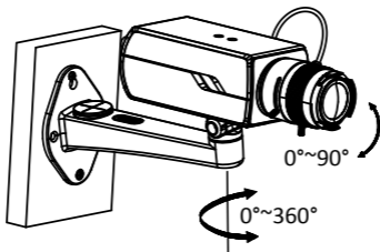
Figura 2-7 Reglați unghiul de supraveghere
